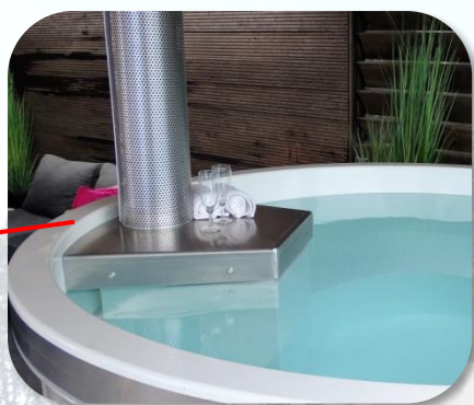
fig. 2 (onderkant tafel) de kachel moet ruim onder water staan, ivm koeling van de kachel en afgifte van warmte
